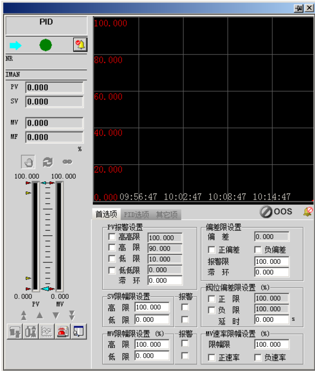
图 2-8 PID功能块的调整画面
