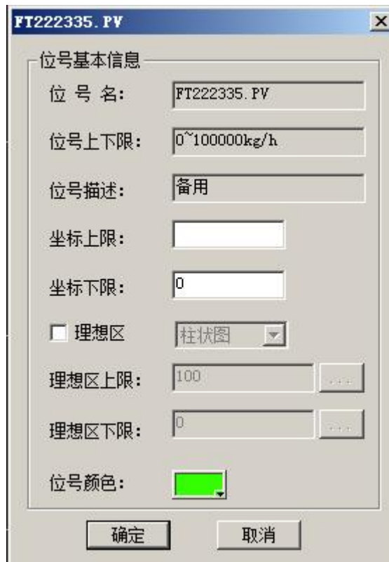
图 1-59 趋势位号属性面板
