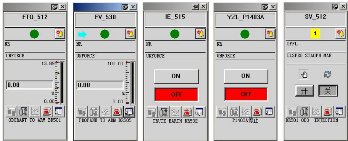
图 1- 8 位号仪表面板 (依次为 AI/AO/DI/DO/开关阀设备)
