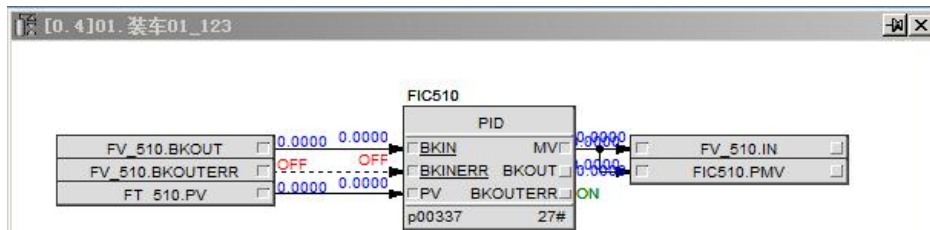
图 1- 9 逻辑图
